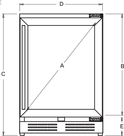
VUE FRONTALE
