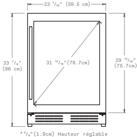
VUE FRONTALE
