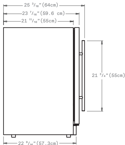
VUE LATÉRALE
