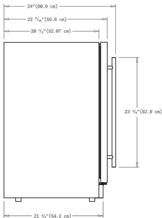
VUE LATÉRALE
