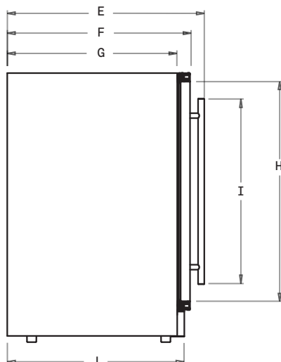
VUE LATÉRALE
