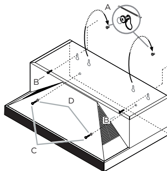
A. Vis de montage B. Vis de sécurité supérieures (Installation al mur) C. Vis de sécurité inférieures (Installation al mur) D. Rondelles
