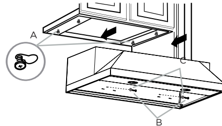
A. 4 vis de montage B. Vis de sécurité C. Rondelles
