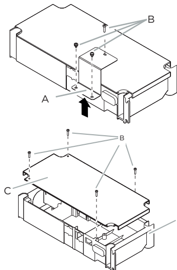
A. Estufa B. Tornillos de la caja de terminales C. Cubierta de la caja de terminales D. Caja de terminales
