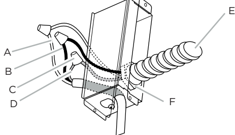
A. Alambres blancos B. Alambres negros C. Conectores de alambres aprobados por UL
